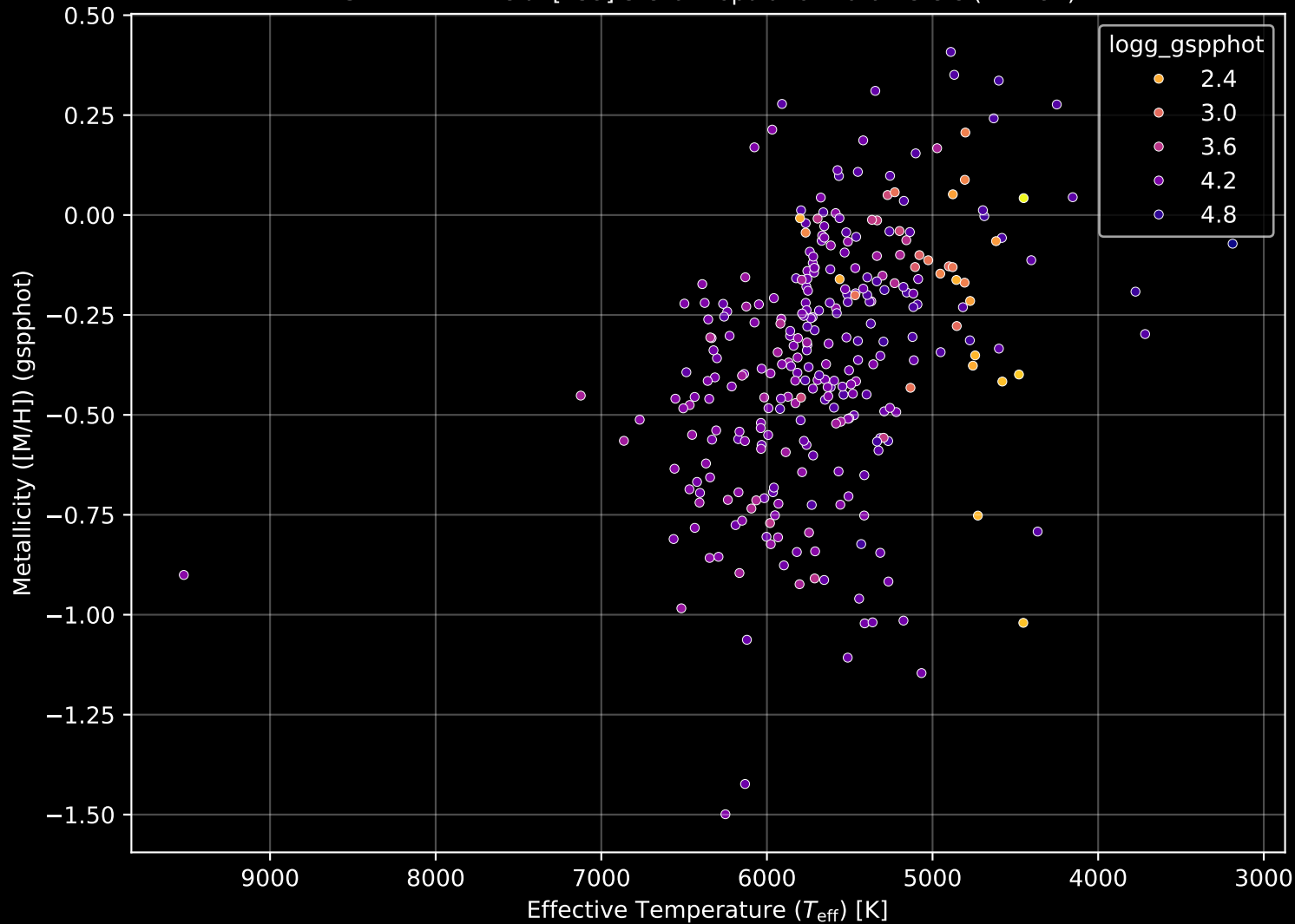
GALAH DR4 Field: [759] Stellar Population Parameters (n= 297)
